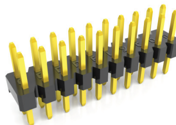
DS1025-05 BARRA DE PINOS 2.0mm 180 GRAUS
