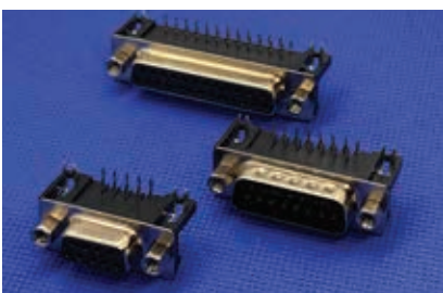
BR5037 CONECTORES DB SOLDA PLACA 90 GRAUS
