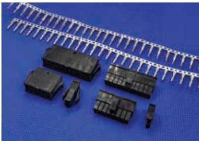
3001 CONECTORES PASSO 3,00 mm (Equivalente ao MICRO FIT)
