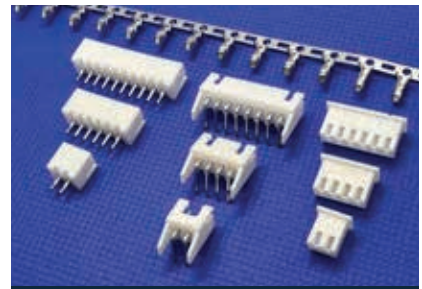
2501 CONECTORES PASSO 2,5 mm (Equivalente JST XH)
