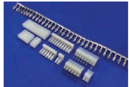
3961 CONECTORES PASSO 3,96 mm (Equivalente ao KK 3,96 mm)
