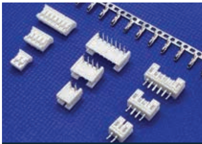
2001 CONECTORES PASSO 2,0 mm (Equivalente JST PH)
